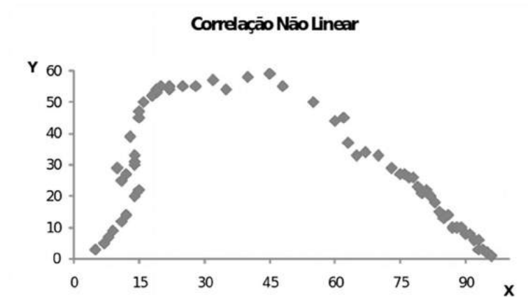
Figura 3.9 Exemplo de correlação não-linear.
