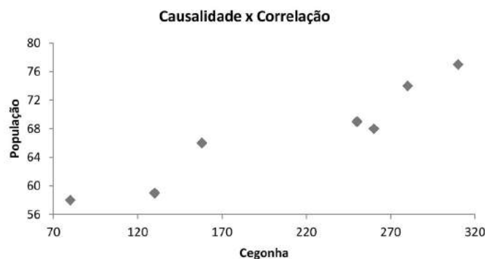
Figura 3.14 Gráfico de dispersão, número de cegonhas versus população da cidade de Oldenberg.
