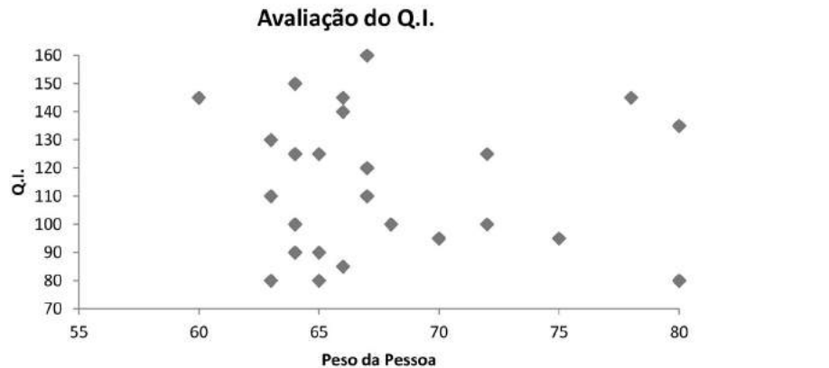
Figura 3.8 Gráfico de dispersão, Q. I. em função do peso da pessoa.
