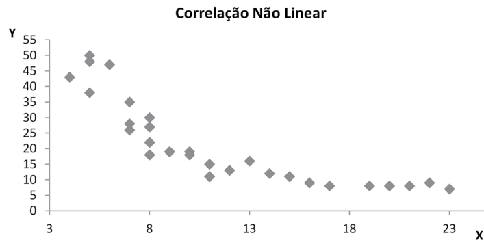
Figura 3.10 Outro exemplo de correlação não-linear.
