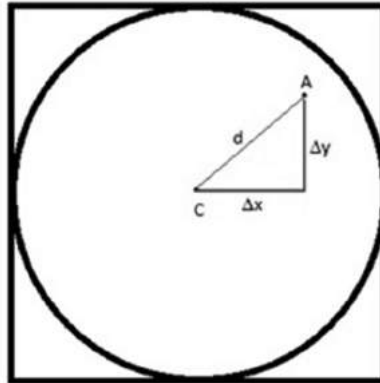
Figura 8.7: Distância d entre qualquer ponto A e o centro da circunferência pode ser calculada através do cálculo de uma hipotenusa.
